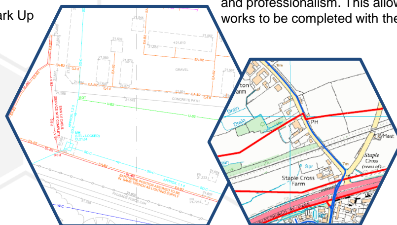
PAS 128 Type B
